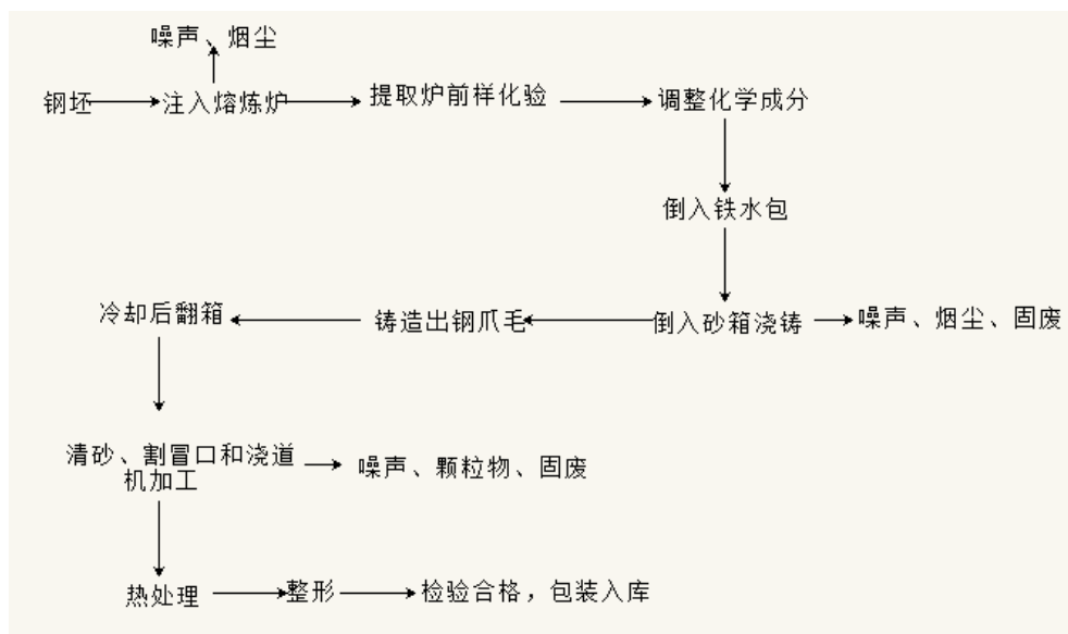
图 3.5-1 生产工艺及产污环节
