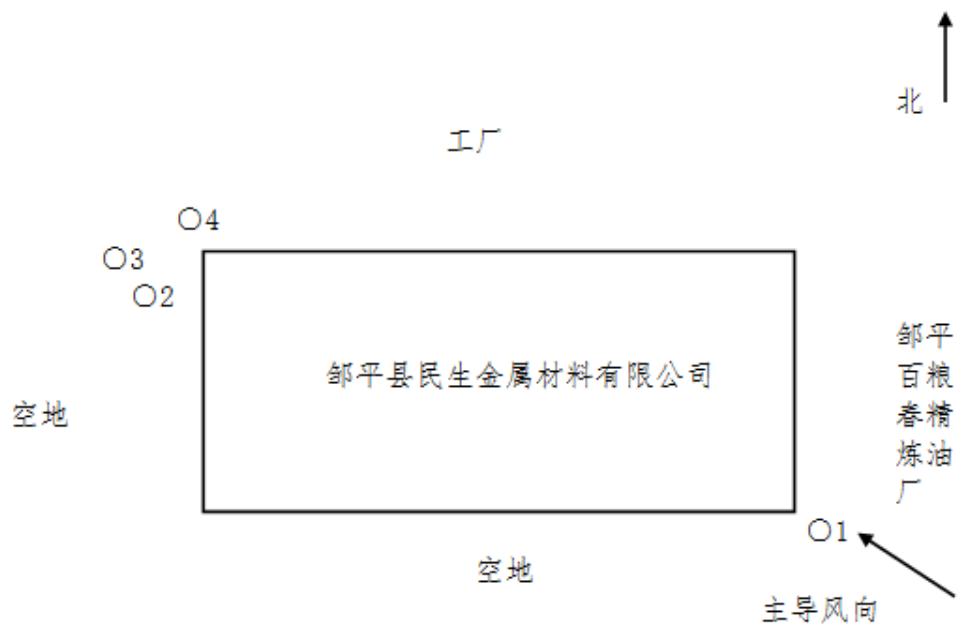
图 7.1-2 该项目厂界无组织废气监测布点图 (2017 年 4 月 13 日) (○表示无组织监测点位)
