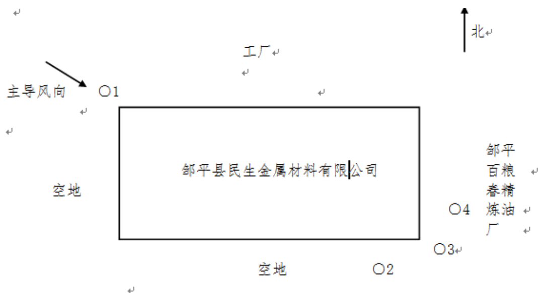
图 7.1-2 该项目厂界无组织废气监测布点图 (2017 年 10 月 23 日~24 日) (○表示无组织监测点位)
